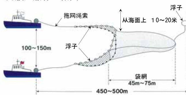
拖网两艘渔船作业概图
