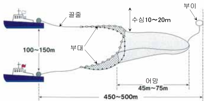
쌍끌이 선인망어선 약도
