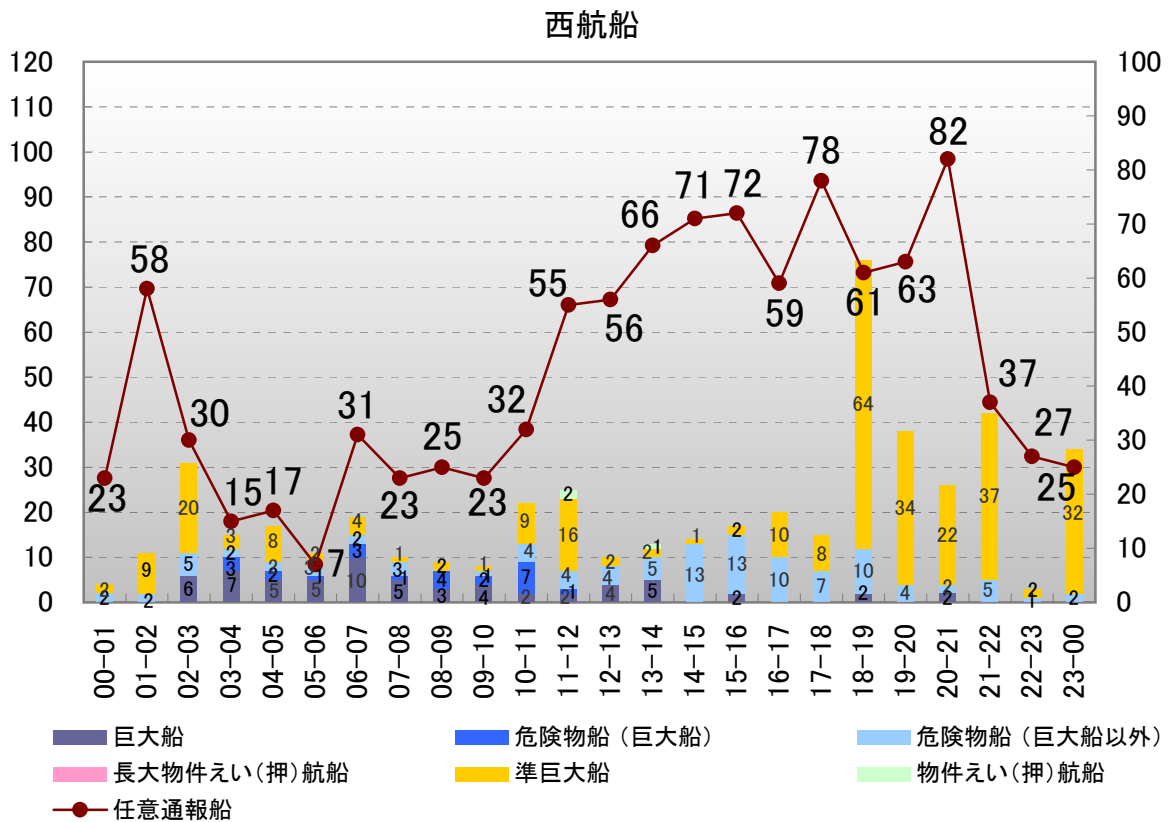
グラフ3-② 時間帯別航路通航隻数
