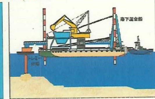
【土砂改良投入作業状況図】 【別件工事】 東亜・青木V
